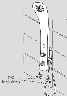
11. Una vez instalada se puede operar con su monomando ó mezcladoras existentes.
