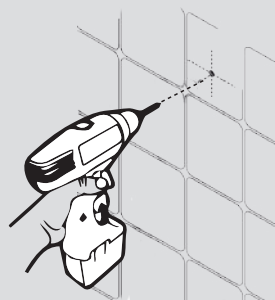
3. Marque y taladre las perforaciones para nuestras bases en el muro.
