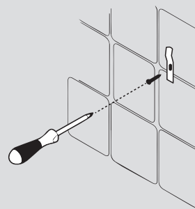
4. Instale taquetes, bases y tornillos (incluidos) en el muro con ayuda de un desarmador de cruz.
